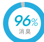
足のニオイなどの元 (イソ吉草酸)
