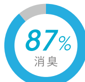
タバコや汗などのニオイの元 (アンモニア)
